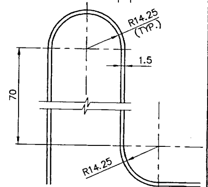
DETAIL - Y
