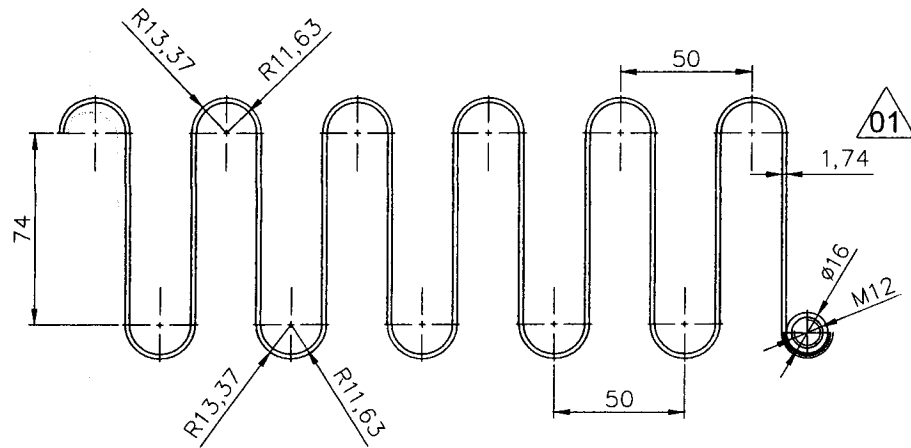
DETAIL-D SCALE-1:2
