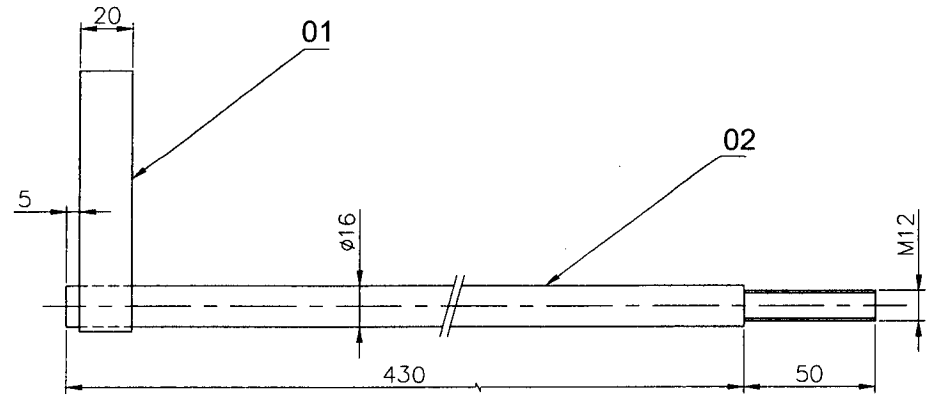
DETAIL-E SCALE-1:2
