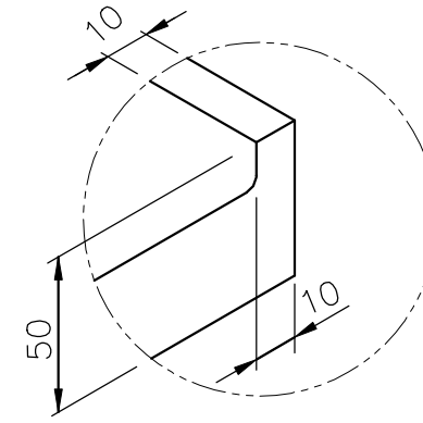
DETAIL-D
