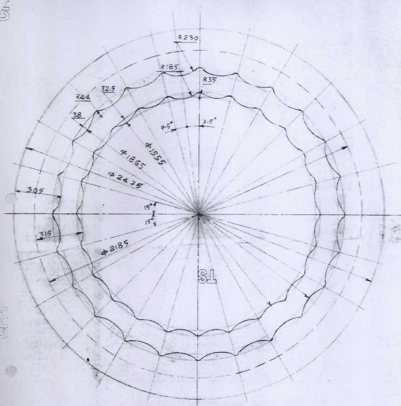
VIEW-A SCALE: 1:10
