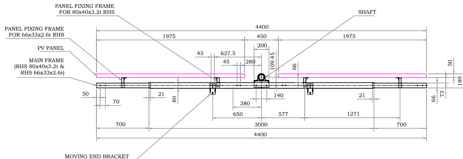
SECTION A-A
