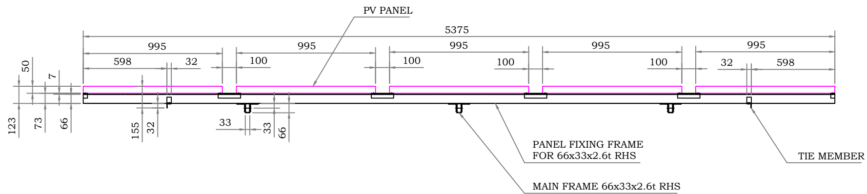
SECTION D-D
