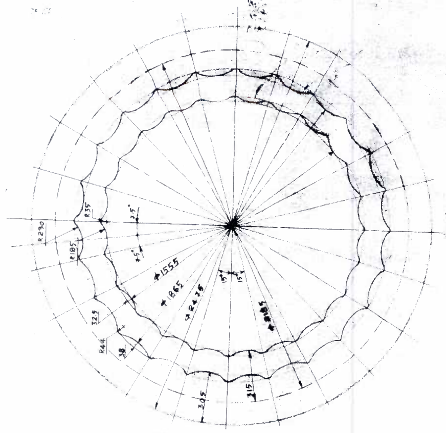
VIEW-A SCALE: 1:10
