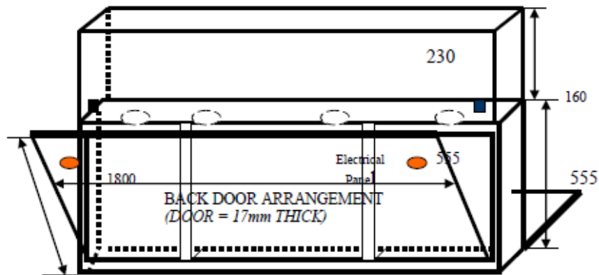
Fig. 1. BACK DOOR ARRANGEMENT
