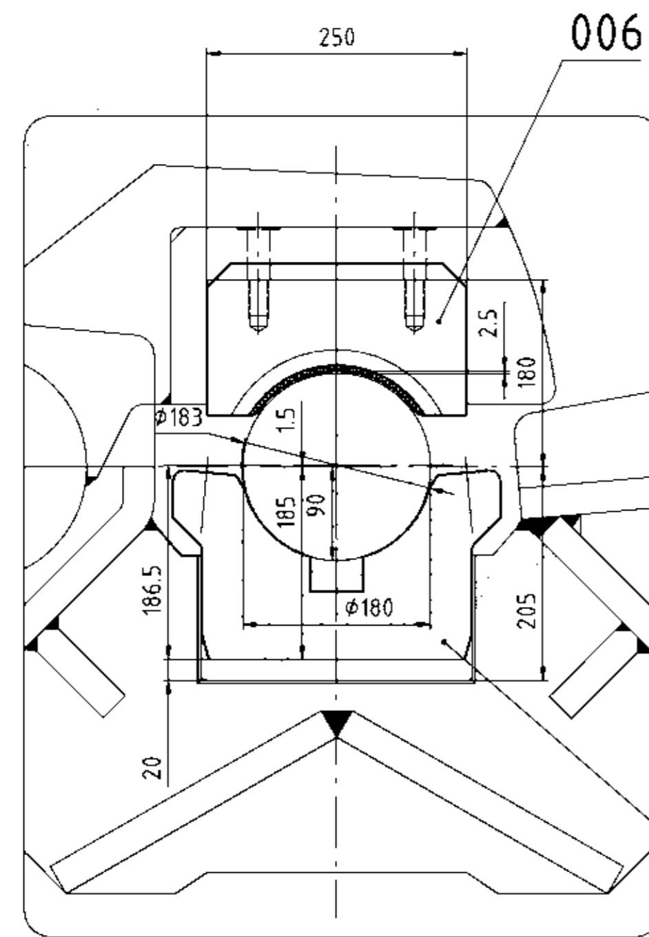
A-A 1:5
