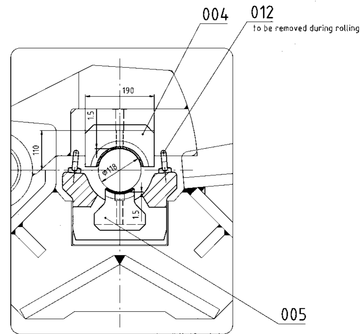
B-B 1:5
