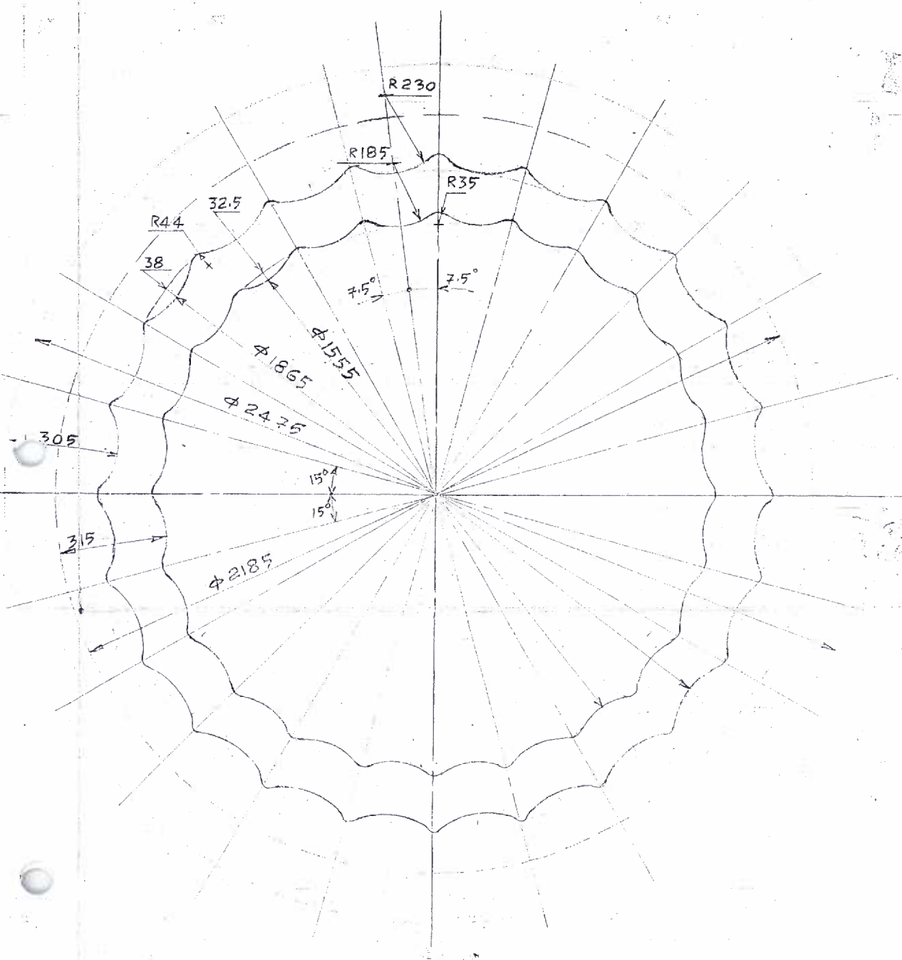
VIEW-A SCALE: 1:10
