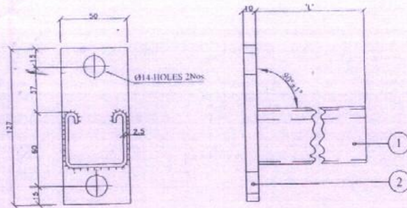
CANTILEVER ARMS
